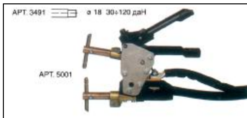
Клещи ручные с воздушным охлаждением. Возможность использования: стандартные плечи и плечи с большим раствором: Арт. 5001...5085.
